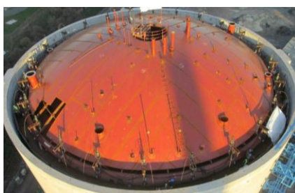
Levage d'un dôme de réservoir Yara Tertre - Belgique
